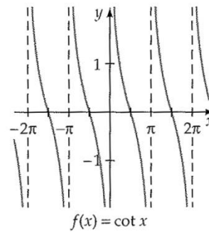
Cotangent function
