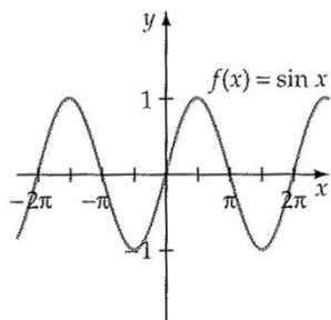
Sine function
